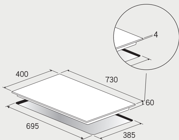
感應爐安裝散熱圖
