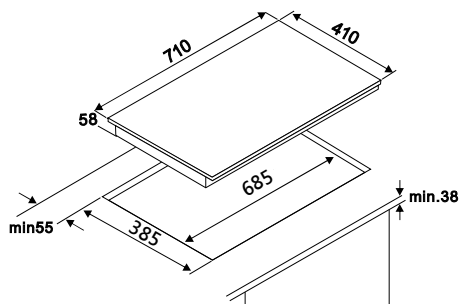
GIH340A 雙口橫式感應爐
