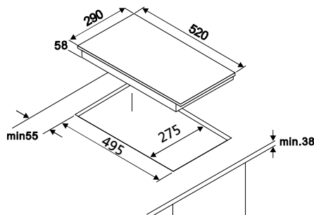
GIO2116 單口感應爐
