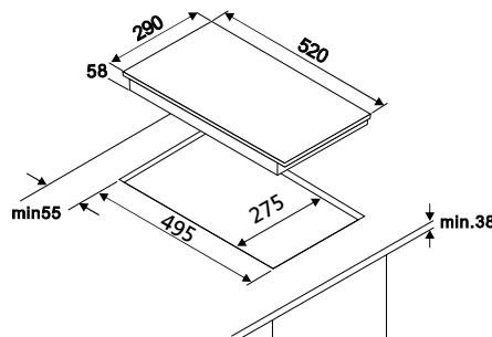
GI3416 雙口感應爐
