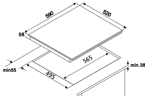
GIT66D04 三口感應爐
