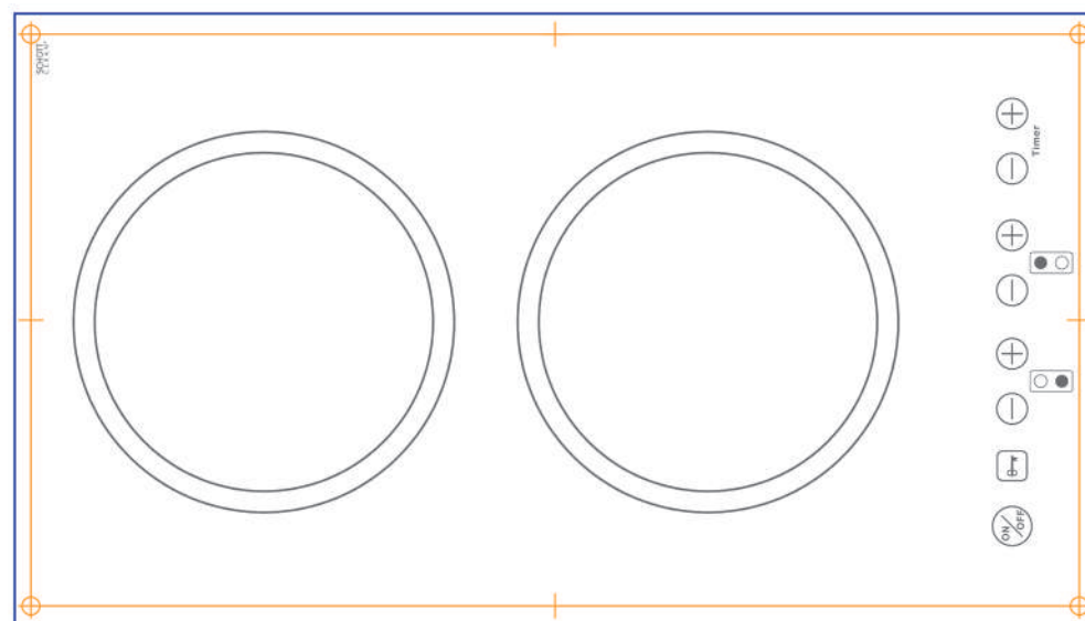
上嵌式挖孔圖 (設備面板高於桌面)
