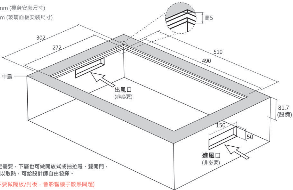
全平式挖孔圖 (設備面板與桌面齊平)
