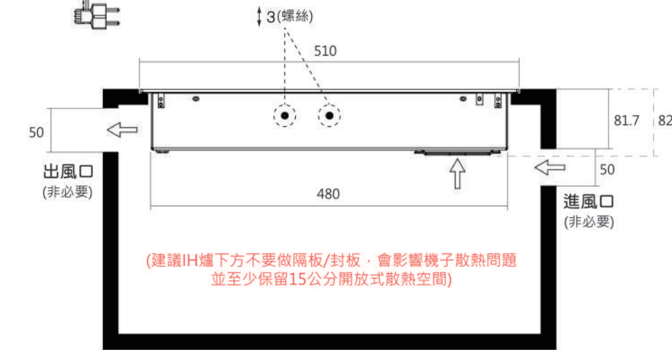
側視圖
