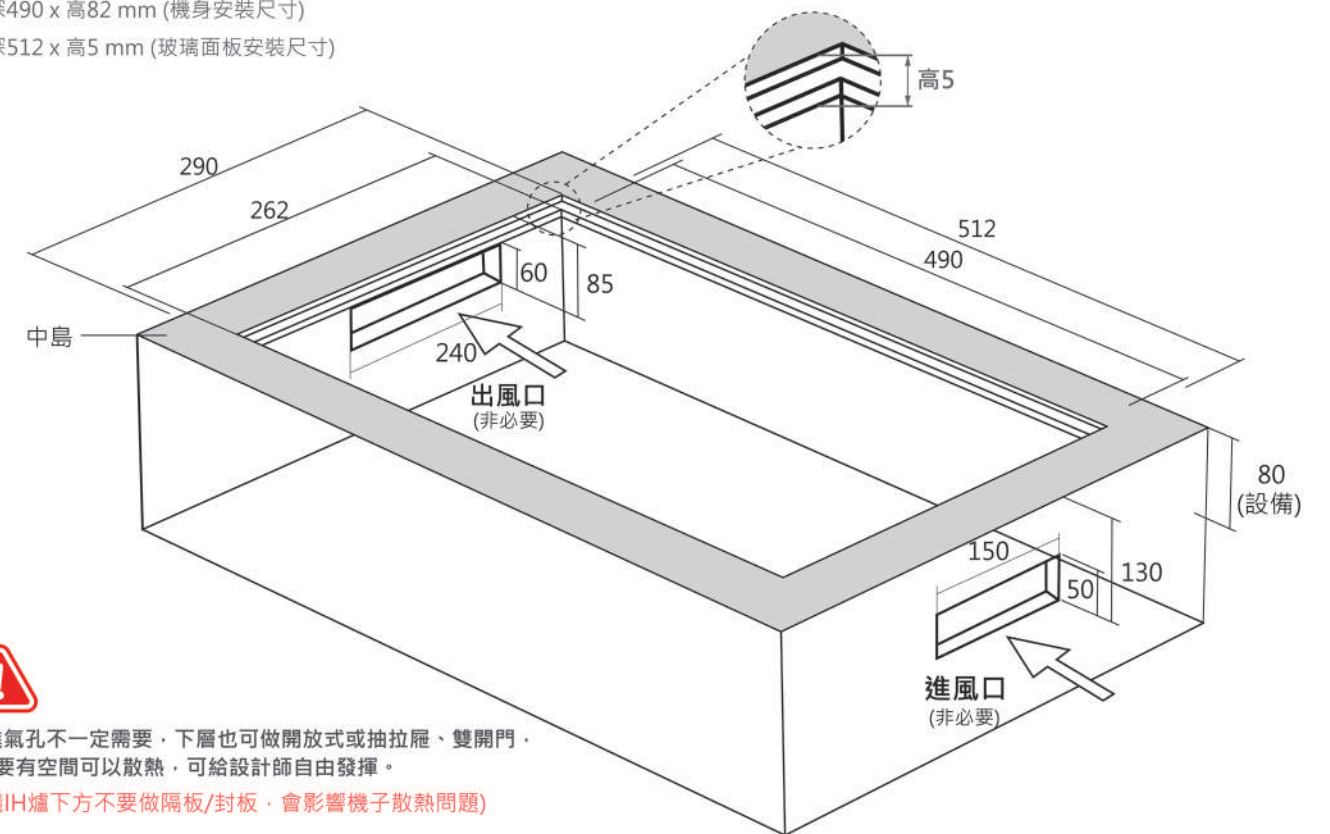
全平式挖孔圖 (設備面板與桌面齊平)
