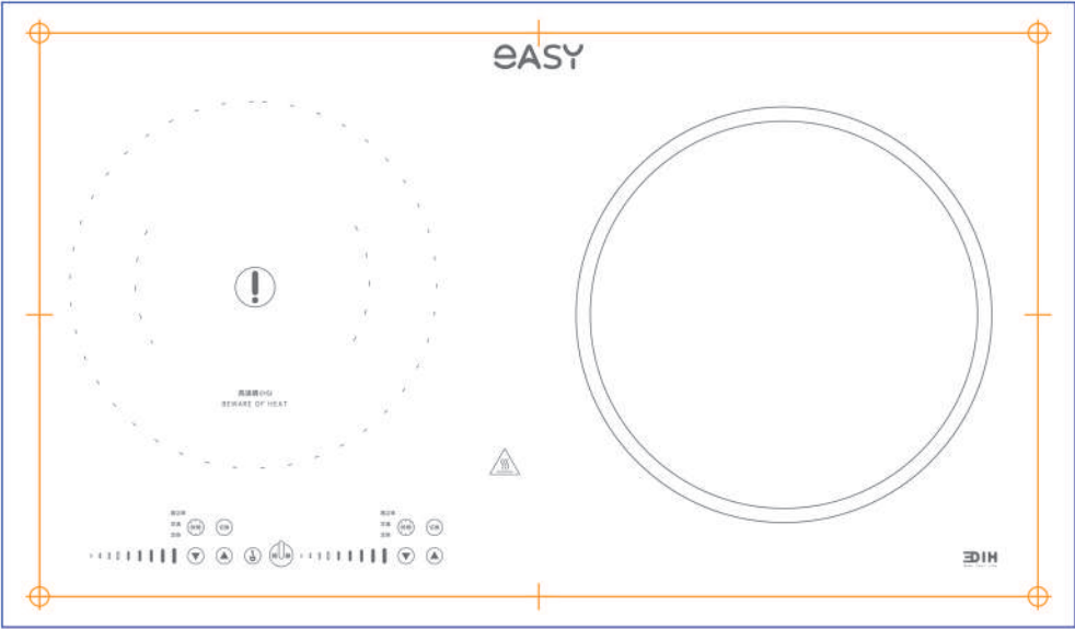
上嵌式挖孔圖 (設備面板高於桌面)
