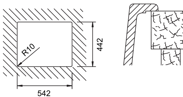
安裝方式：上嵌式開孔
