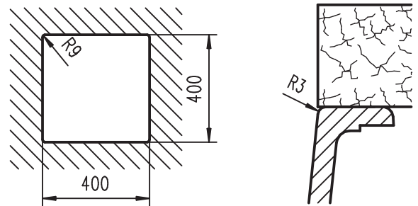
安裝方式：下嵌式開孔
