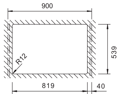
安裝方式：下嵌式開孔
