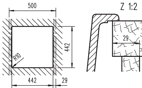
安裝方式：上嵌式開孔
