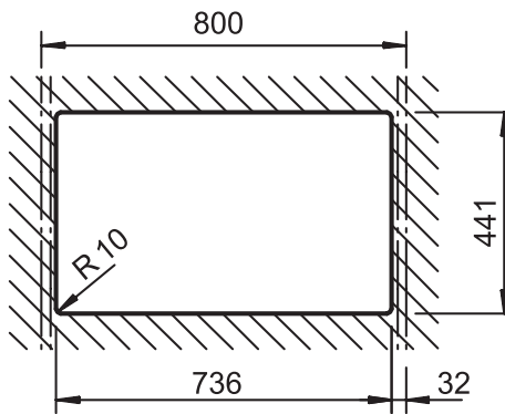
安裝方式：上嵌式開孔
