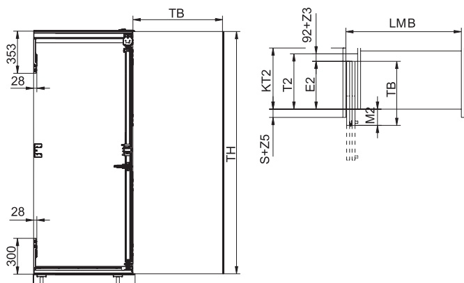
縮回的門扇與外部齊平
