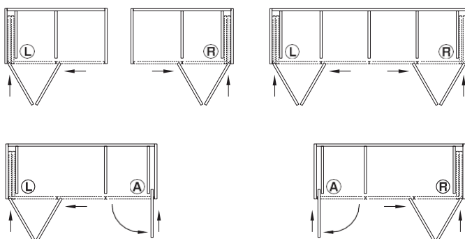
附 1-4 門的櫃式版本
