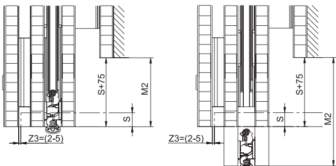
縮回的門扇與外部齊平
