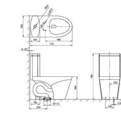
One-Piece Toilet Size : 715x363x780mm Seat : PP Soft-closing Rough-in : 305mm Dual Flush: 3/4.5L Flush System:Siphon 連體座便器 尺寸: 715x363x780mm 蓋板: PP緩降蓋板 坑距: 305mm 名義用水量: 3/4.5L 沖水系統:虹吸
