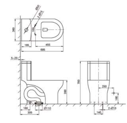
One-Piece Toilet Size : 685x360x700mm Cover Seat : PP Soft-closing Rough-in : 305mm Dual Flush: 3/4.5L Flush System:Siphon 連體座便器 尺寸: 685x360x700mm 蓋板: PP緩降蓋板 坑距: 305mm 名義用水量: 3/4.5L 沖水系統:虹吸
